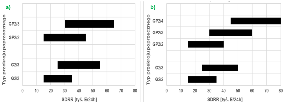
Rys. 5.2.3. Wartości granicznych natężeń ruchu dla poszczególnych typów przekroju wielojezdniowej drogi głównej ruchu przyspieszonego (GPs) i drogi głównej (Gs) ze skrzyżowaniami z sygnalizacją świetlną: a) w obszarach zamiejskich; b) w obszarach miejskich
