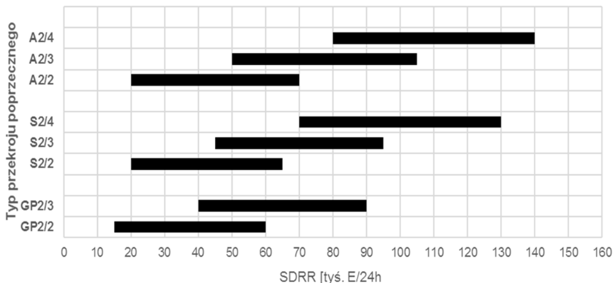
Rys. 5.2.1. Wartości granicznych natężeń ruchu dla poszczególnych typów przekroju wielojezdniowej autostrady (A), drogi ekspresowej (S) i drogi głównej ruchu przyspieszonego z węzłami (GPw) w obszarach zamiejskich.
