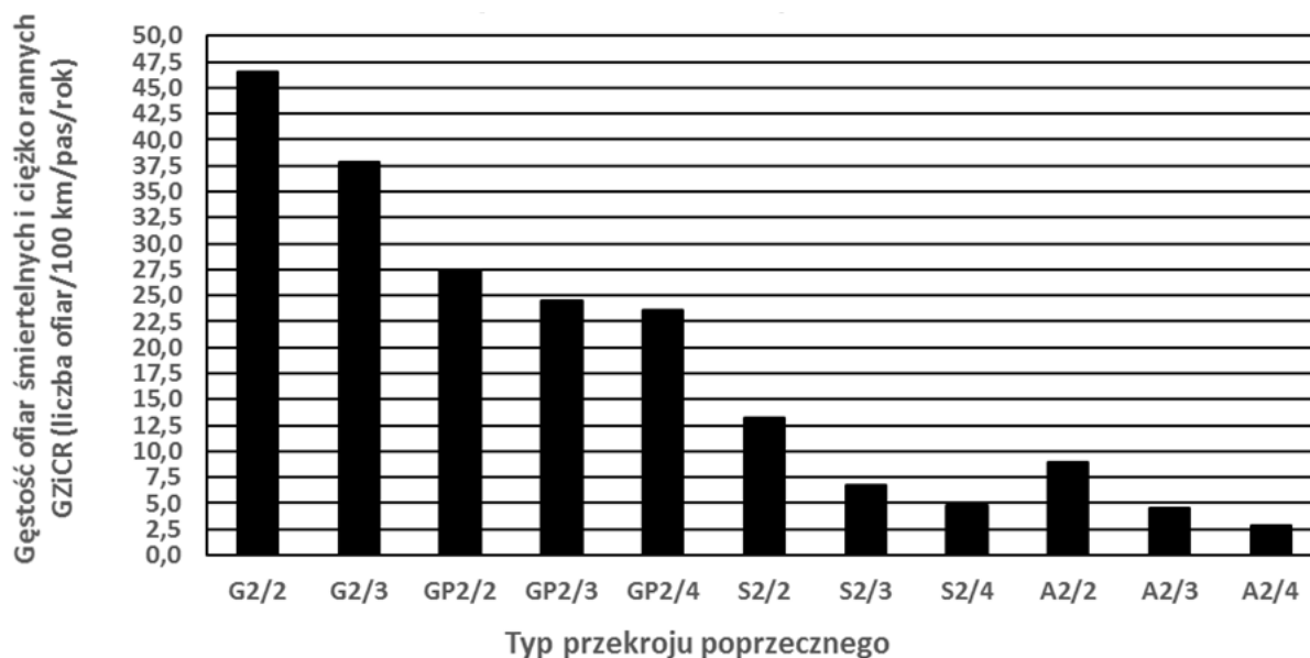
Rys. 5.2.4. Wykres rozkładu średnich gęstości ofiar śmiertelnych i ciężko rannych liczonych dla 100 km odcinka drogi w zależności od zastosowanego typu przekroju poprzecznego drogi
