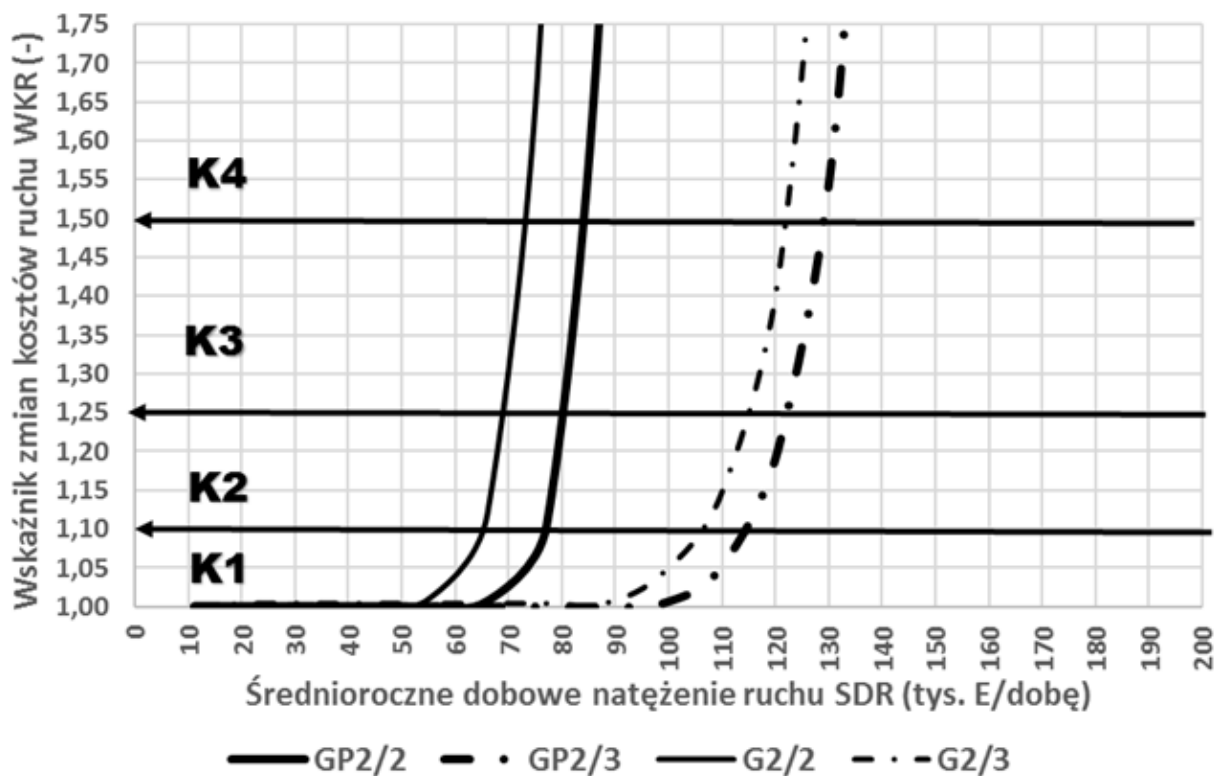
Rys. 5.2.8. Wykresy zmienności wskaźnika zmian kosztów drogowych i kosztów ruchu WKR na wzorcowym odcinku drogi głównej ruchu przyspieszonego lub drogi głównej w zależności od zastosowanego typu przekroju poprzecznego drogi
