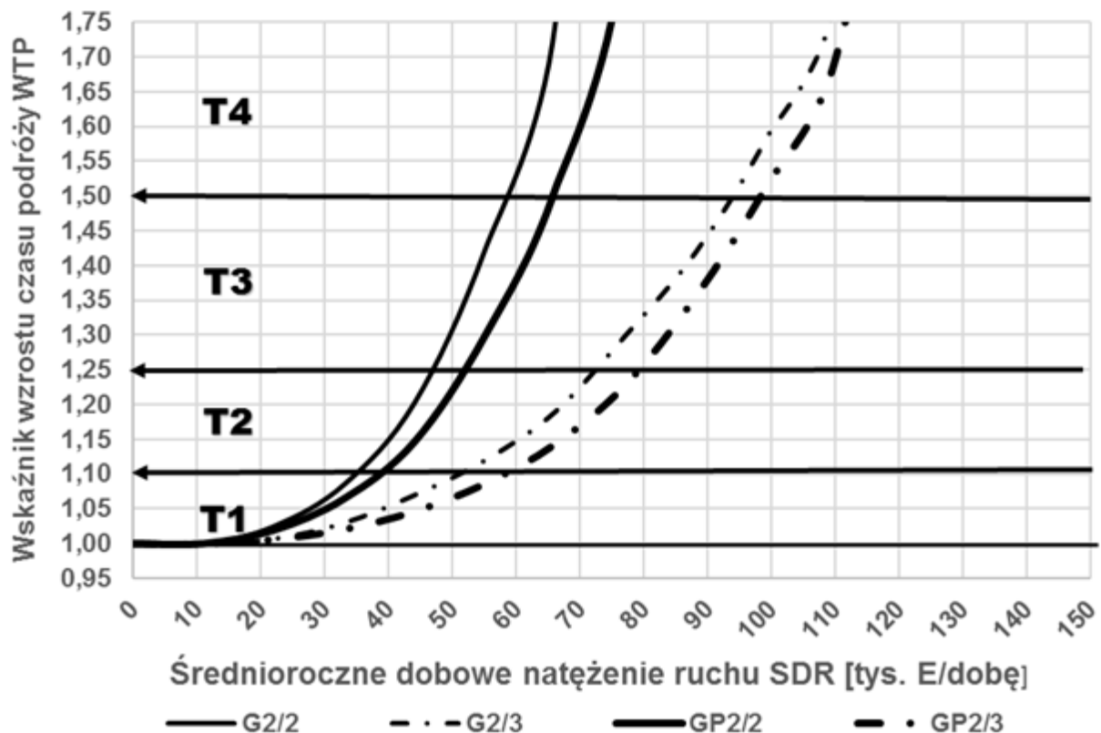
Rys. 5.2.6. Wykres zmienności wskaźnika wydłużenia czasu podróży WTP na wzorcowym odcinku drogi głównej ruchu przyspieszonego lub drogi głównej w zależności od zastosowanego typu przekroju poprzecznego drogi
