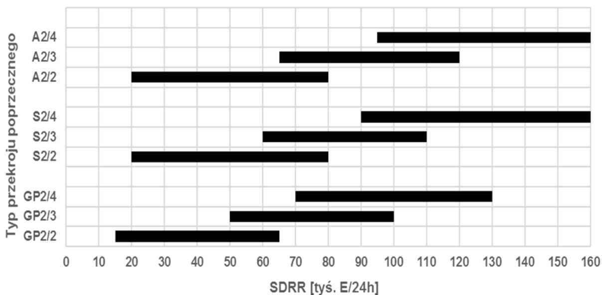
Rys. 5.2.2. Wartości granicznych natężeń ruchu dla poszczególnych typów przekroju wielojezdniowej autostrady (A), drogi ekspresowej (S) i drogi głównej ruchu przyspieszonego z węzłami (GPw) w obszarach aglomeracji miejskich.
