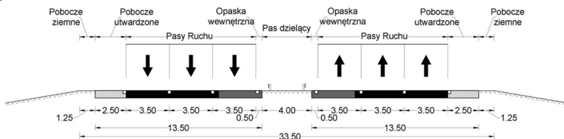
Rys. 4.2.3.1. Schemat przedstawiający realizację scenariusza SE 2 rozbudowy przekroju poprzecznego drogi
