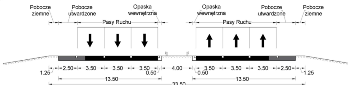
Rys. 4.2.3.2. Schemat przedstawiający realizację scenariusza SE 3 rozbudowy przekroju poprzecznego drogi
