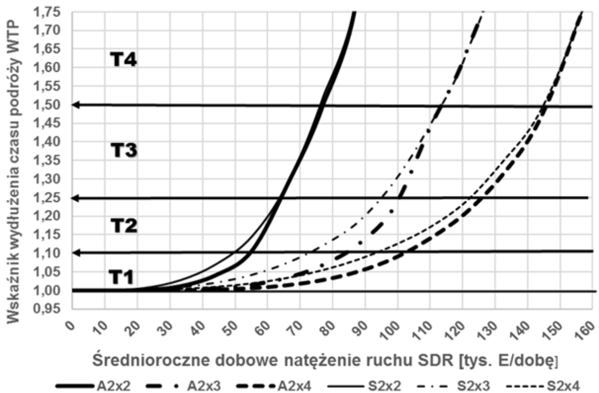
Rys. 5.2.5. Wykres zmienności wskaźnika wydłużenia czasu podróży WTP na wzorcowym odcinku autostrady lub drogi ekspresowej w zależności od zastosowanego typu przekroju poprzecznego drogi
