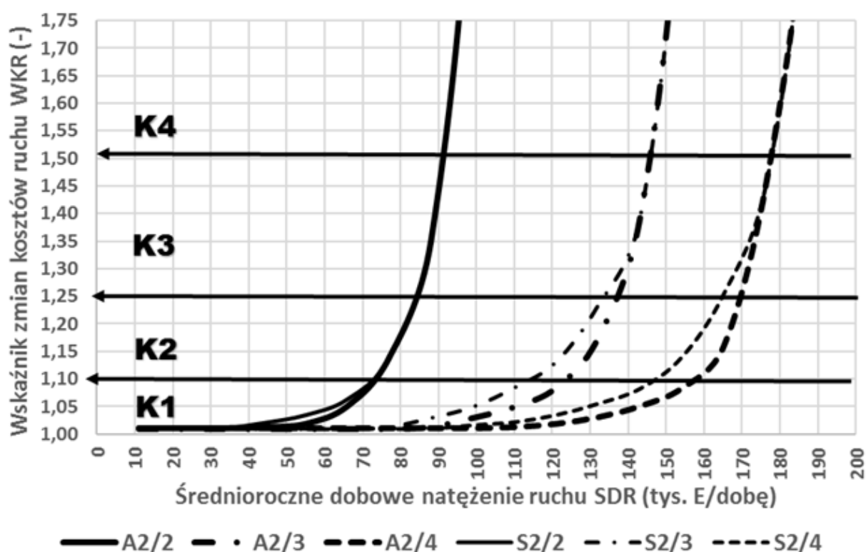
Rys. 5.2.7. Wykresy zmienności wskaźnika zmian kosztów drogowych i kosztów ruchu WKR na wzorcowym odcinku autostrady lub drogi ekspresowej w zależności od zastosowanego typu przekroju poprzecznego drogi
