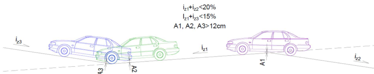
Rys. 8.3.1. Kształtowanie pochyień podłużnych zjazdu przy dużych spadkach
