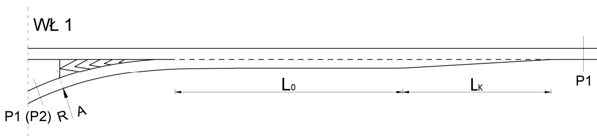
Rys. 9.3.4.1. Schemat typowego rozwiązania wjazdu z równoległym pasem włączania
